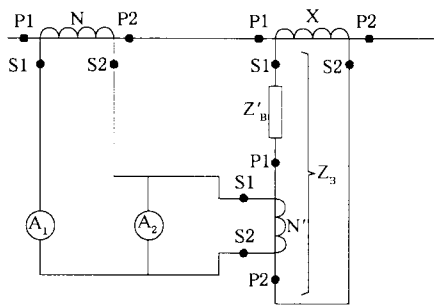
图 2D.6 另一种试验电路
