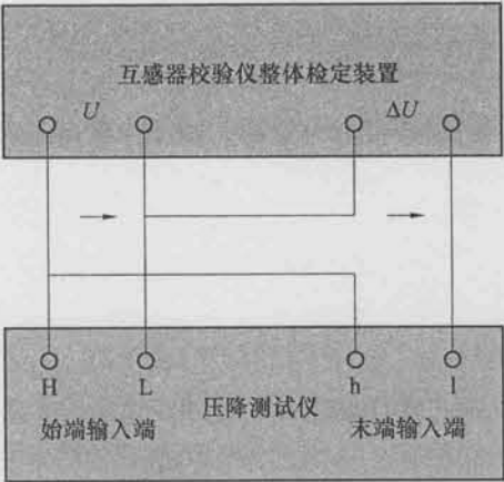
图4 基本误差试验接线图
