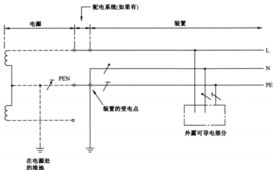
图 7.1.1 - 6 在装置的受电点将 PEN 分离成 PE 和 N 的单相 2 线制的 TN-C-S 系统
