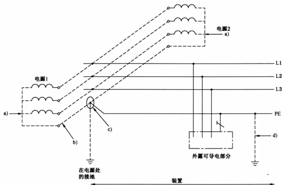
图 7.1.1-9 给 2 相或 3 相负荷供电的全系统内只有 PE 没有 N 的多电源 TN 系统
