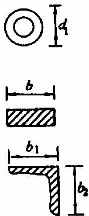
图 A.0.1-2 几种型式导体的计算用尺寸
