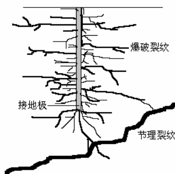
图 9 单根垂直接地极采用深孔爆破接地技术后形成的填充了降阻剂的区域
