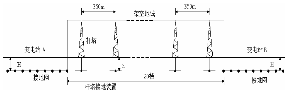
图 11 变电站 A 发生内部接地故障
