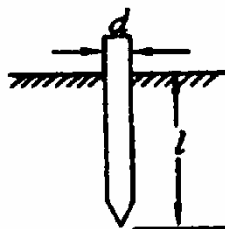
图 A.0.1-1 垂直接地极的示意
