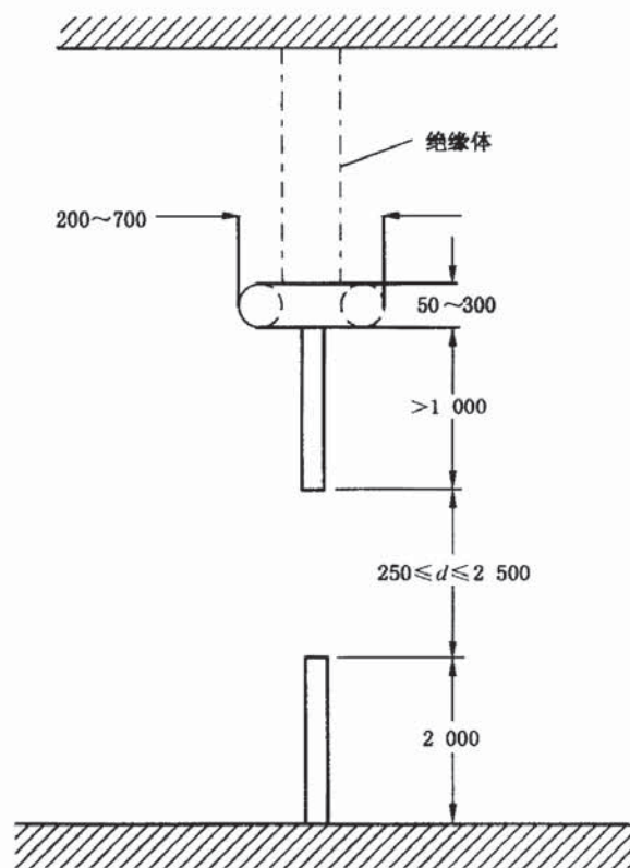
a) 垂直布置
