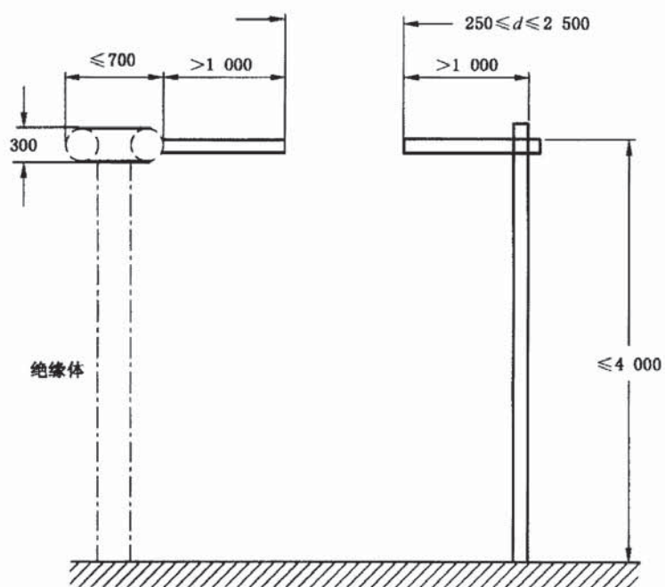
b) 水平布置
