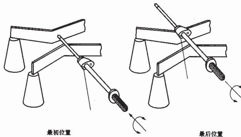
图 9 桥式保护，试验步骤 2
