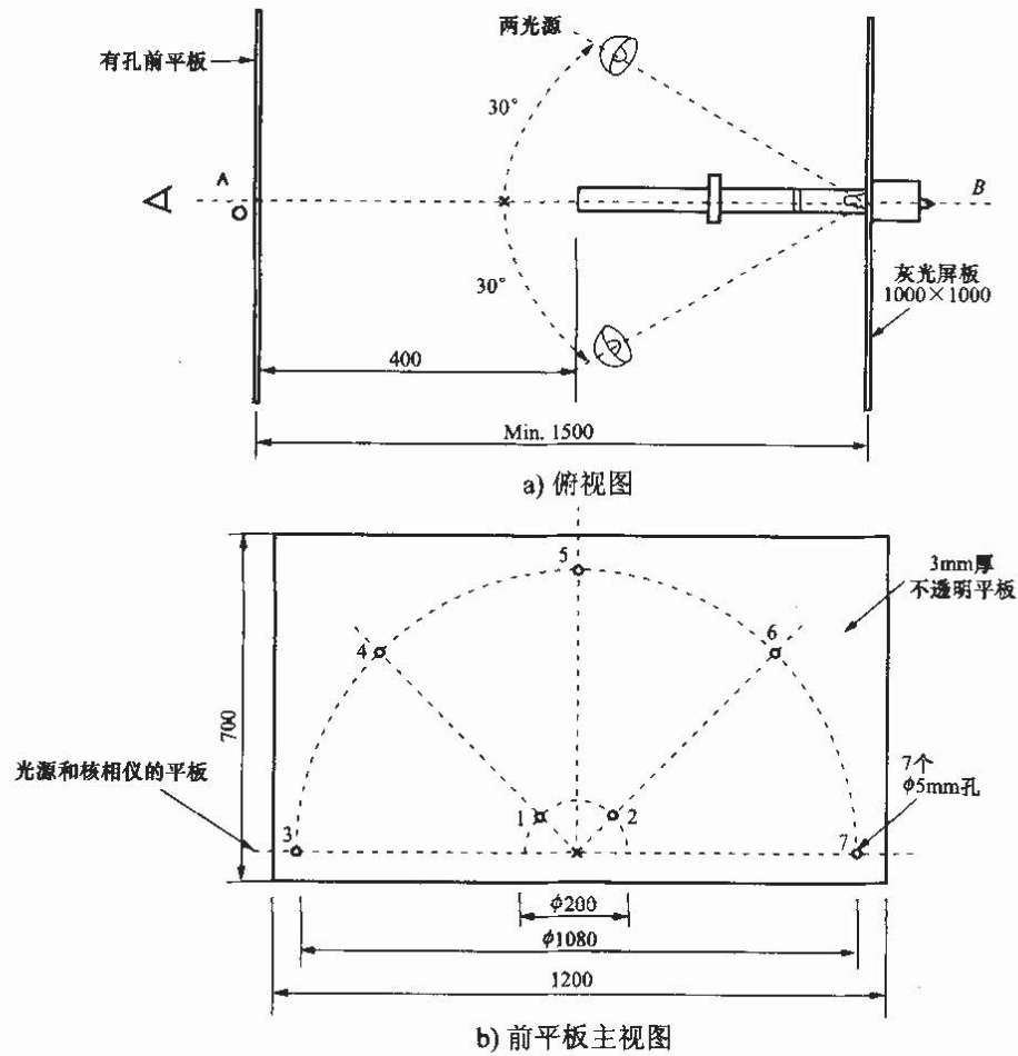
图 4 可视指示易感觉的试验布置
