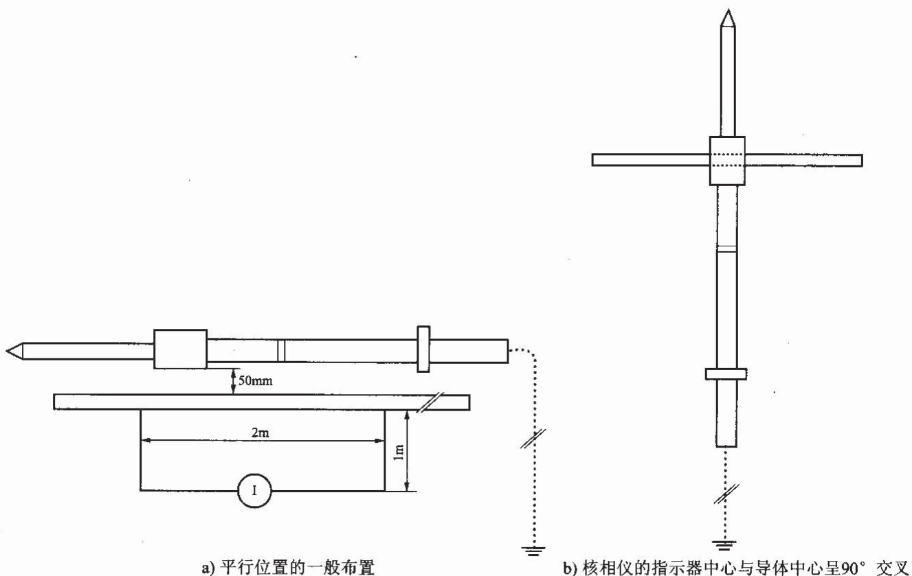
图 3 磁场干扰的影响试验布置
