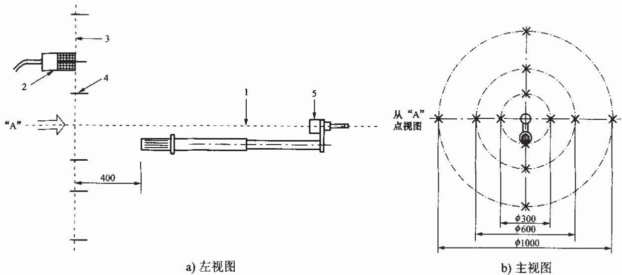
图 4 可视指示易感觉的试验布置
