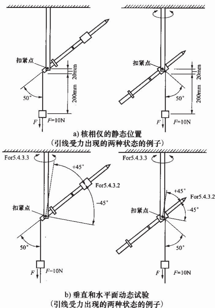
图 12 引线 and 连接强度试验布置
