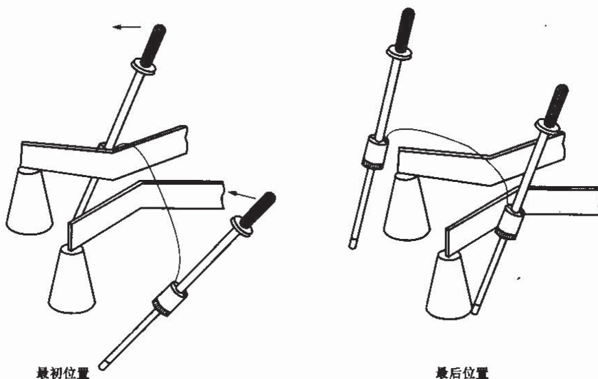
图 10 桥式保护，试验步骤 3
