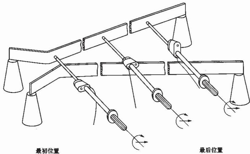
图 7 桥式保护，试验步骤 1
