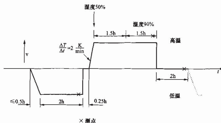
图 13 耐气候电阻循环试验曲线
