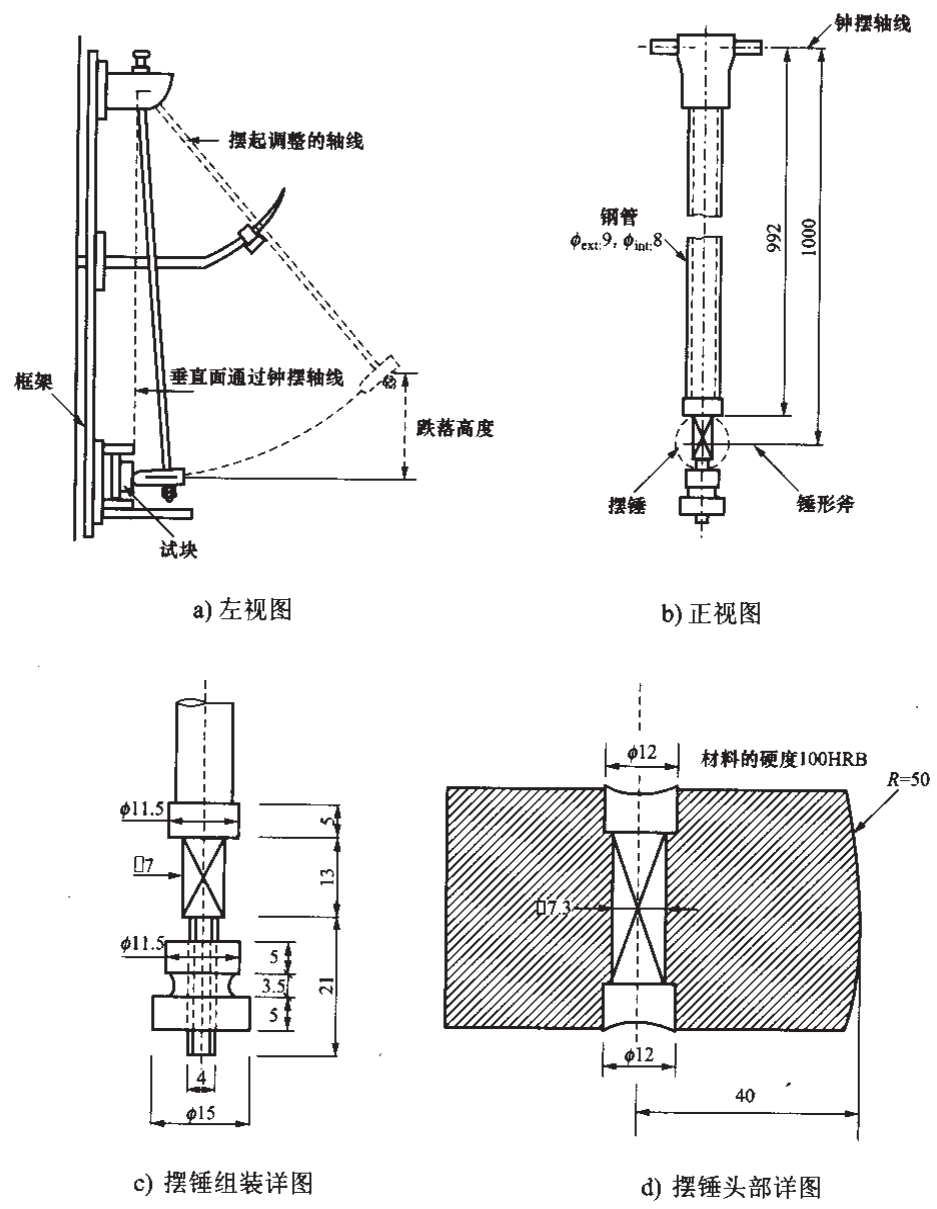
机械性冲击试验——摆锤法
